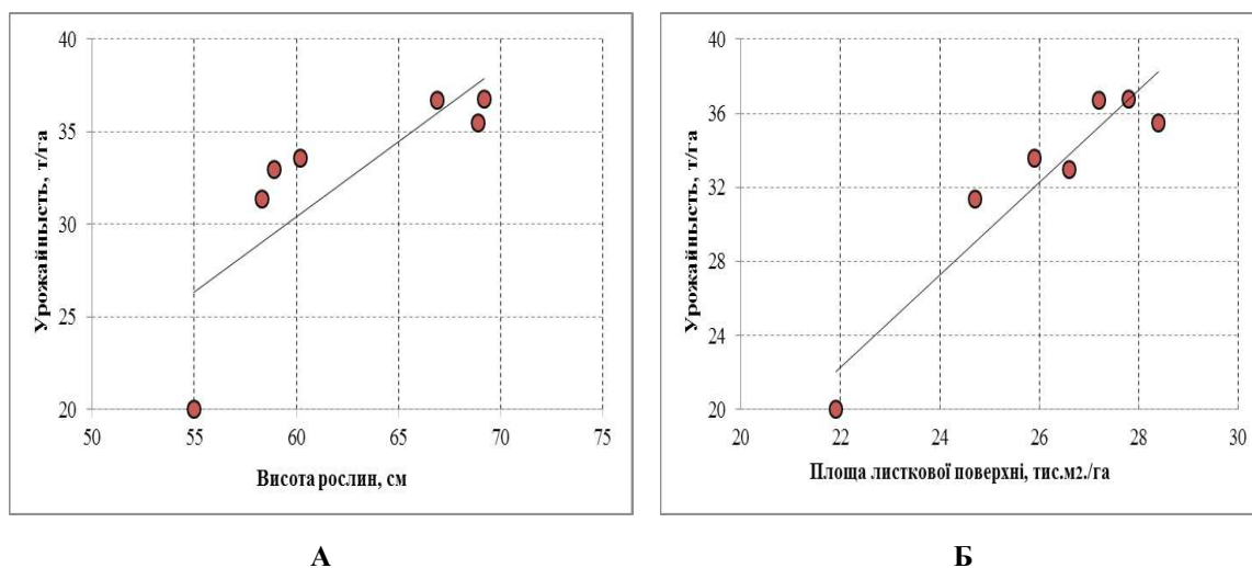
Рис. 1. Кореляційна залежність урожайності картоплі від висоти рослин (А) та площі листкової поверхні (Б).
